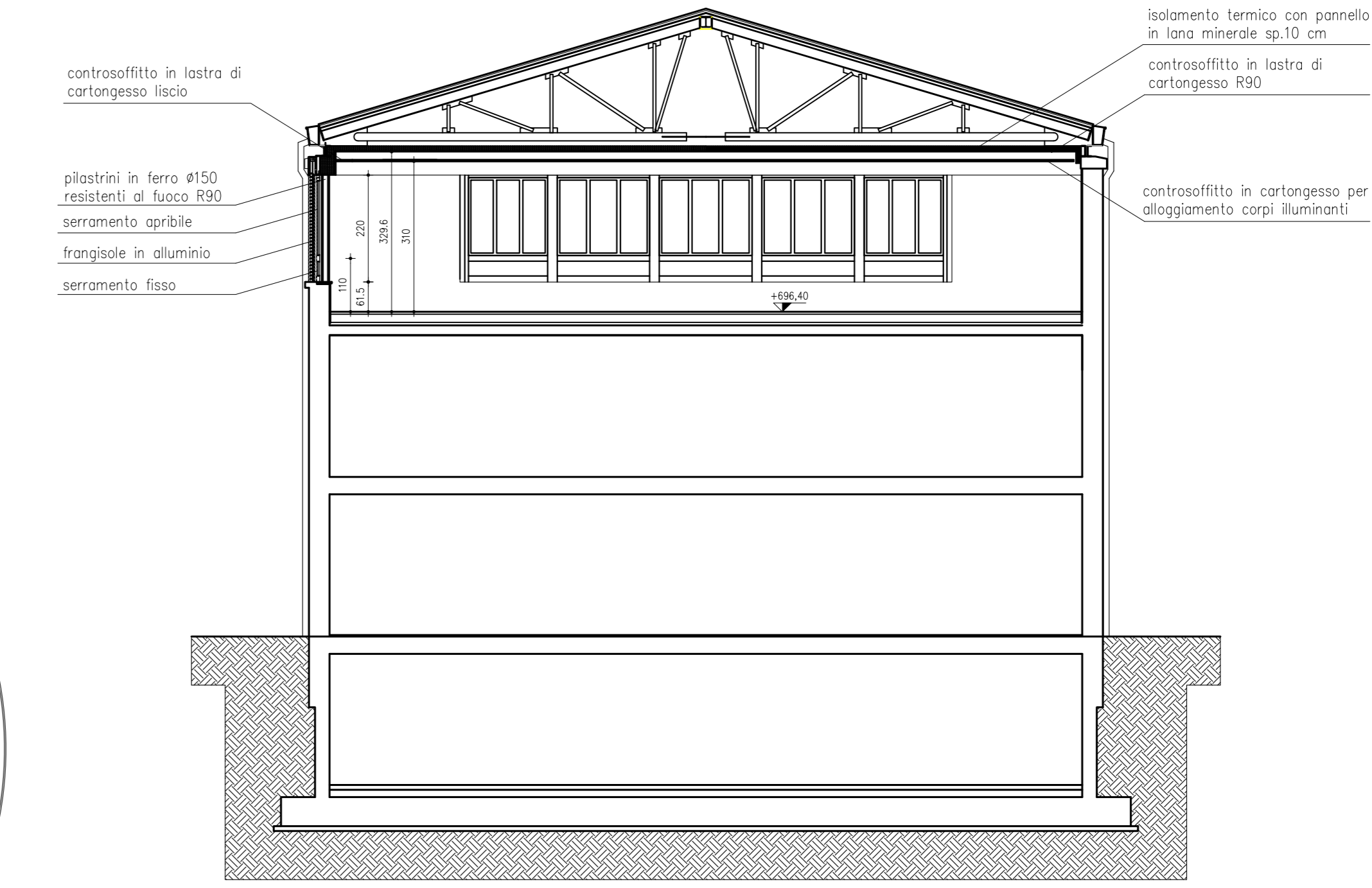
STATO FUTURO - TORRE R/O SEZIONE X-X
