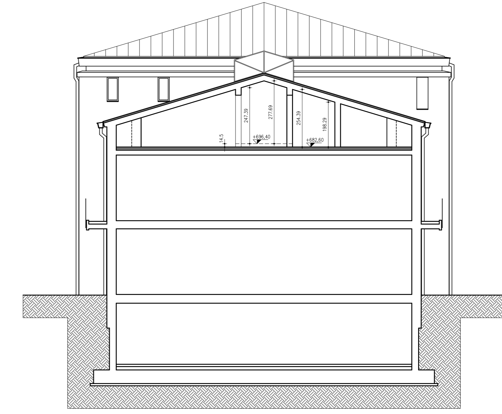
STATO FUTURO - NUCLEO R VISTA DA SUD - SEZIONE Y-Y
